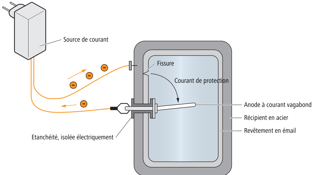
Fig. 17: Anode à courant vagabond (schéma: Blickle, Technique d'installation)
