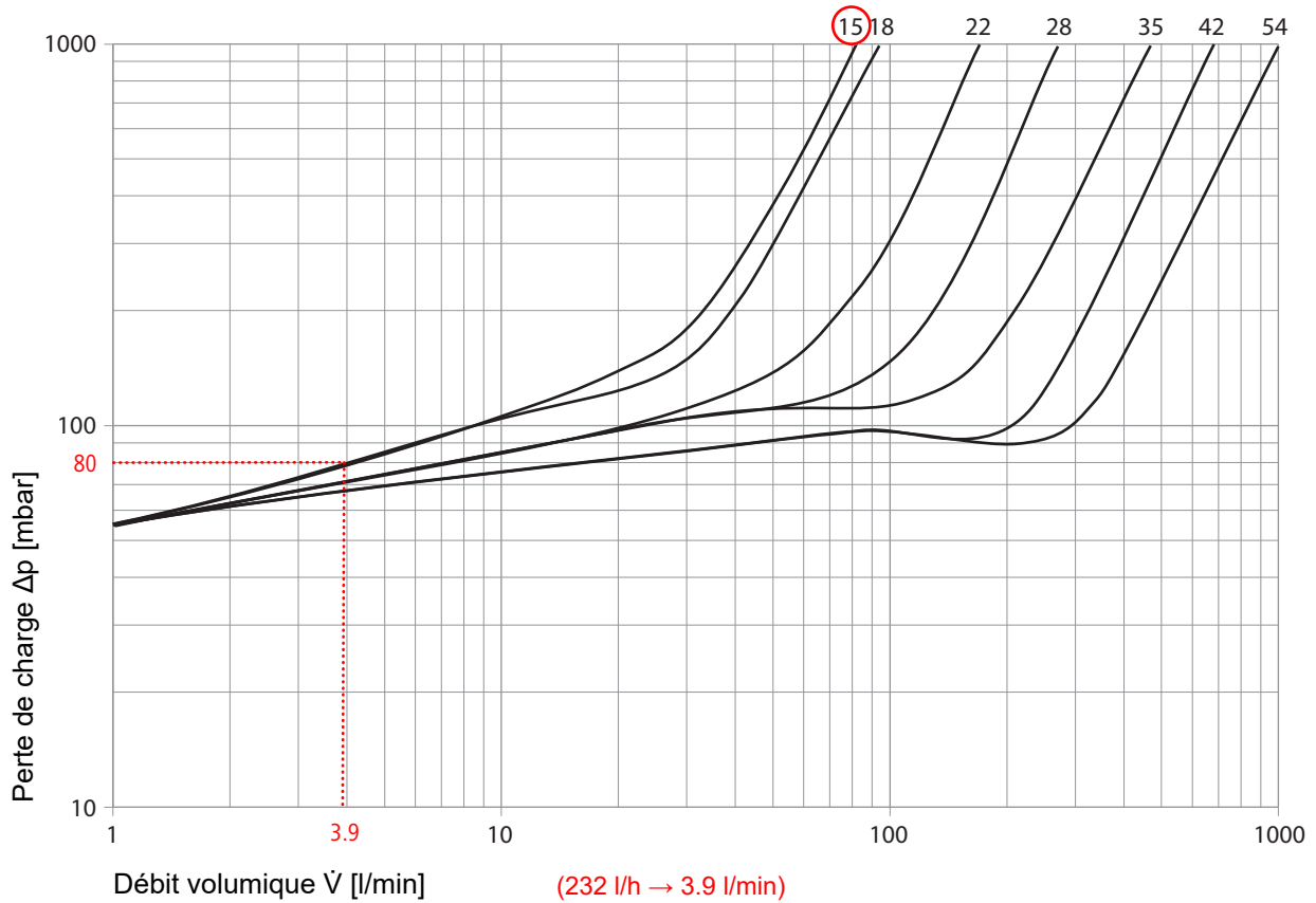
Fig. 46: Clapet anti-retour Optipress-Aquaplus 80189/81163: exemple de lecture du diagramme de performance
