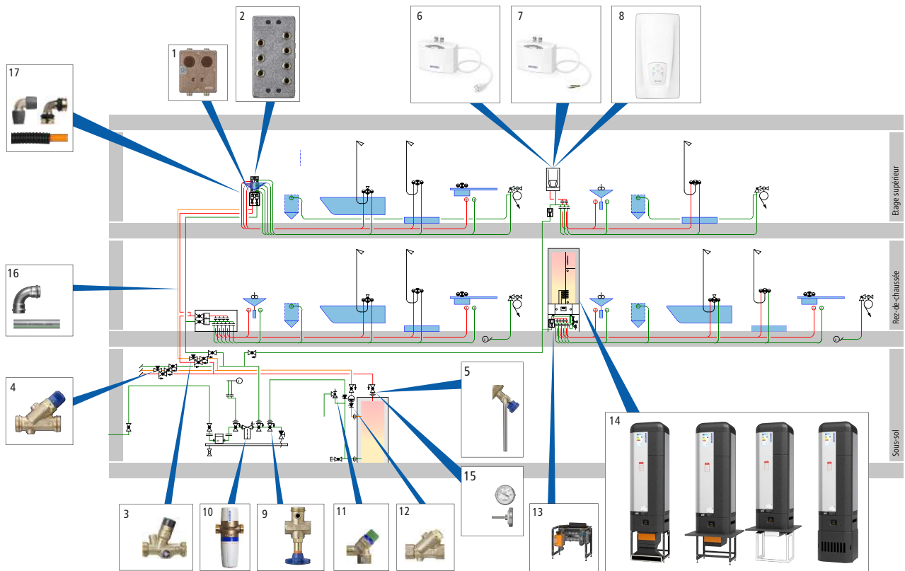
Fig. 45: Solutions Nussbaum pour l’approvisionnement en eau chaude
