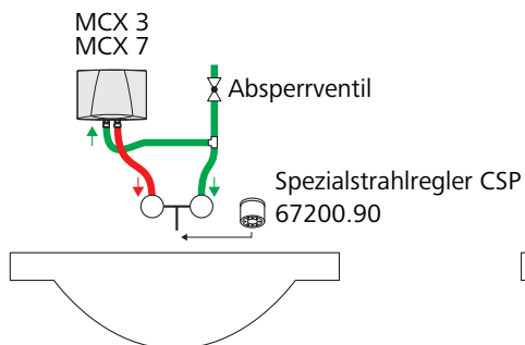
Abb. 2: Montagebeispiel Übertischmontage
