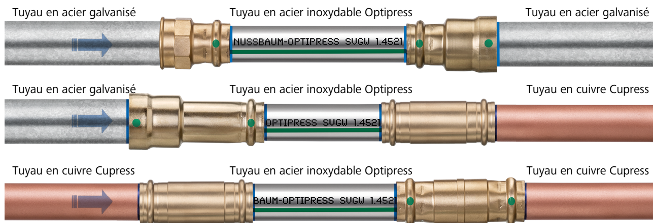
Fig. 4: Installations mixtes admissibles avec Optipress-Aquaplus
