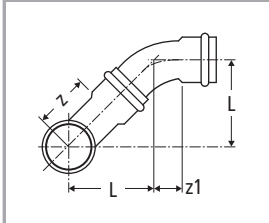
Combinazione Optipress-Gaz 88000 / 88004
