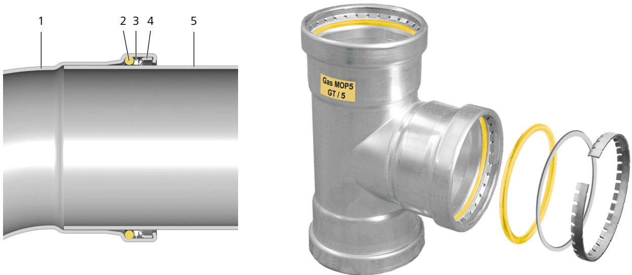
Fig. 2: Raccordo a pressione Optipress-Gaz XL Ø 64,0, 76,1, 88,9 e 108,0 mm
