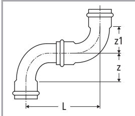
Combinazione Optipress-Gaz 88000 / 88001
