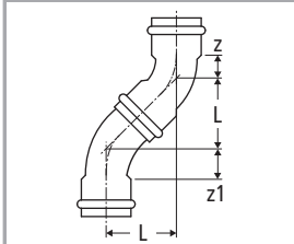
Combinazione Optipress-Gaz 88003 / 88004
