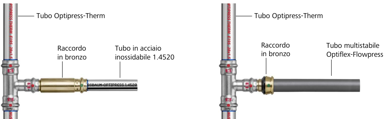
Fig. 3: Installazioni miste consentite di Optipress-Therm su Optipress-Aquaplus e Optiflex-Flowpress
