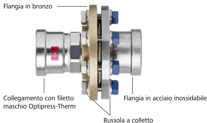
Fig. 3: Installazioni miste consentite di Optipress-Therm su Optipress-Aquaplus e Optiflex-Flowpress
