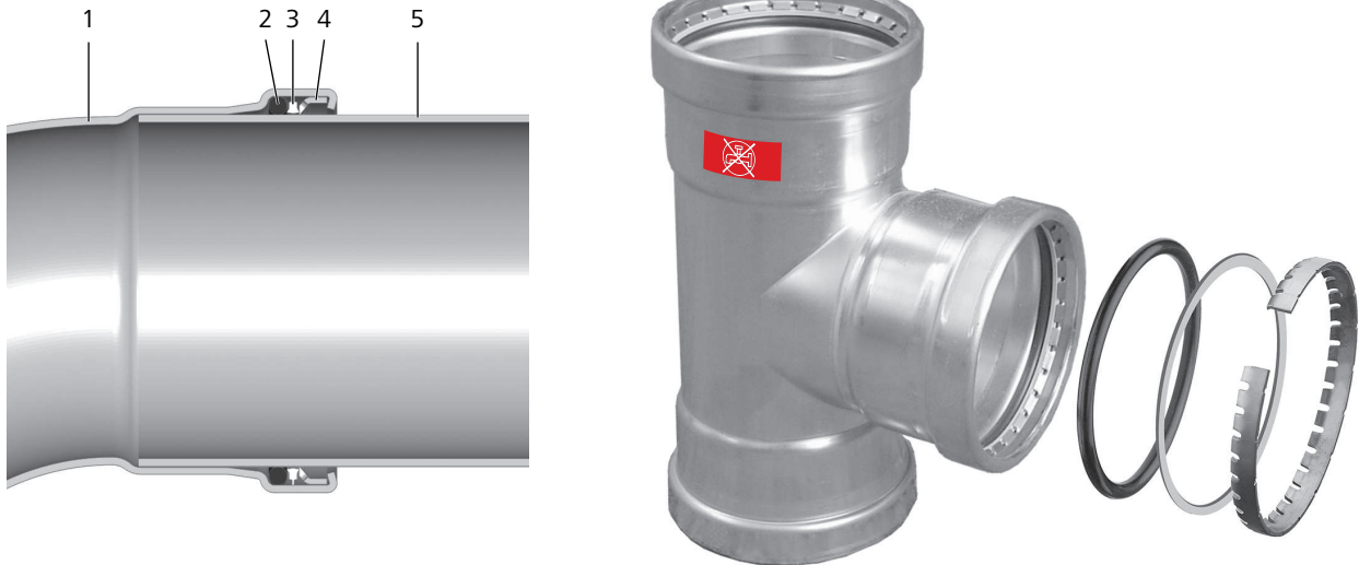
Fig. 2: Raccordo a pressione Optipress-Therm XL Ø 64, 76.1, 88.9 e 108 mm
