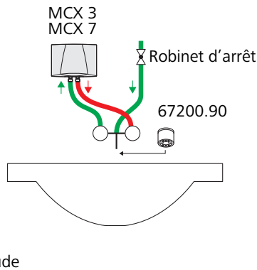
Fig. 2: Exemple de montage pour un montage sur lavabo
