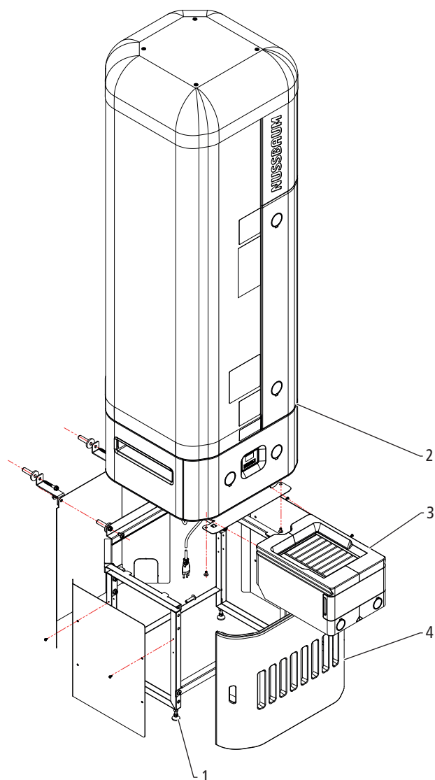
Fig. 1: 68030 Chauffe-eau pompe à chaleur Aquapro-Ecotherma, installation libre
