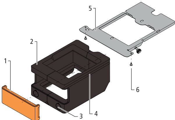
Fig. 5: Corps du filtre à air (sans filtre à air) 68013 et rail de guidage 68967
