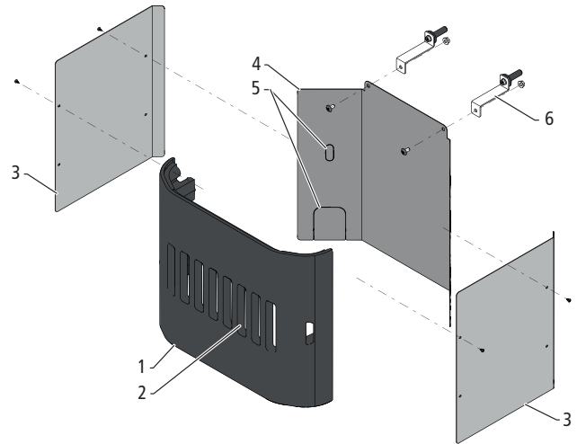
Fig. 6: Couvercle de soubassement 68031
