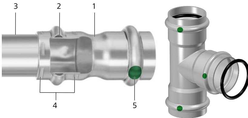
(1) Fitting, (2) Dichtring, (3) Rohr, (4) Doppelte Verpressung, (5) Kennzeichnung SC-Contour
