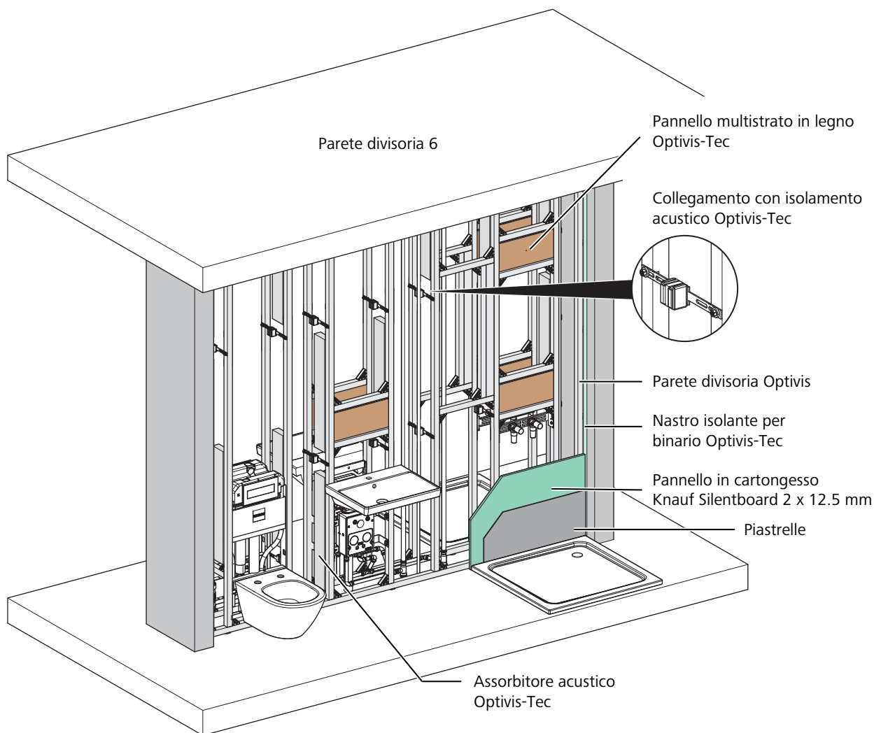
Fig. 35: Parete divisoria Optimis 34.5 cm, con rivestimento su entrambi i lati
