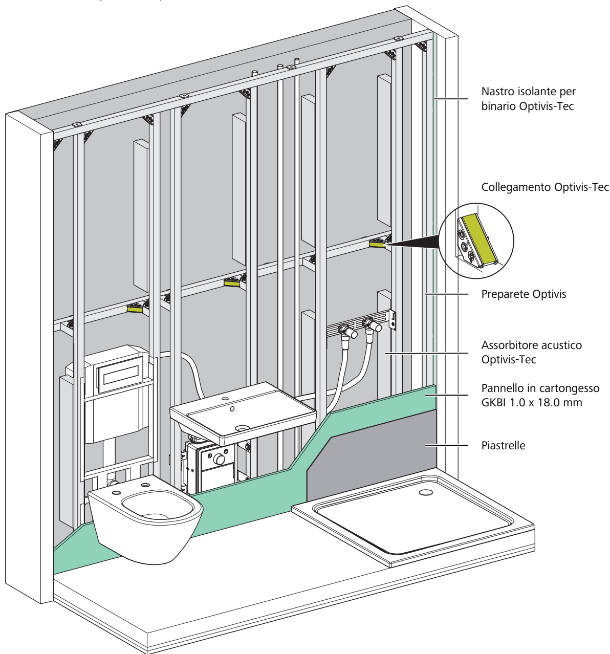
Fig. 15: Componenti idrosanitari preparete Optivis
