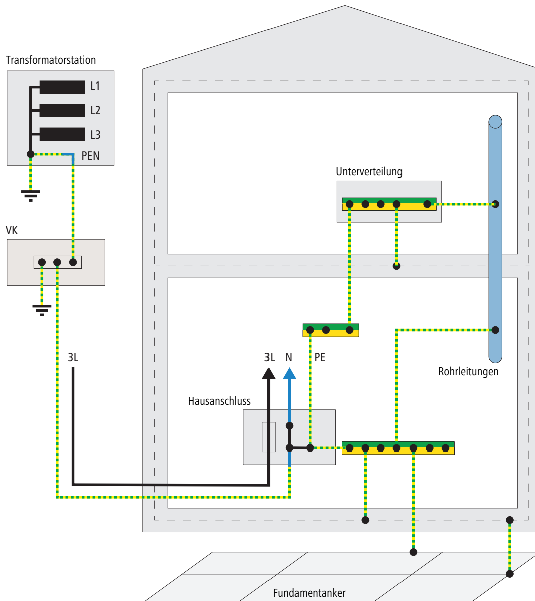
Abb. 27: TN-C-Netzsystem
