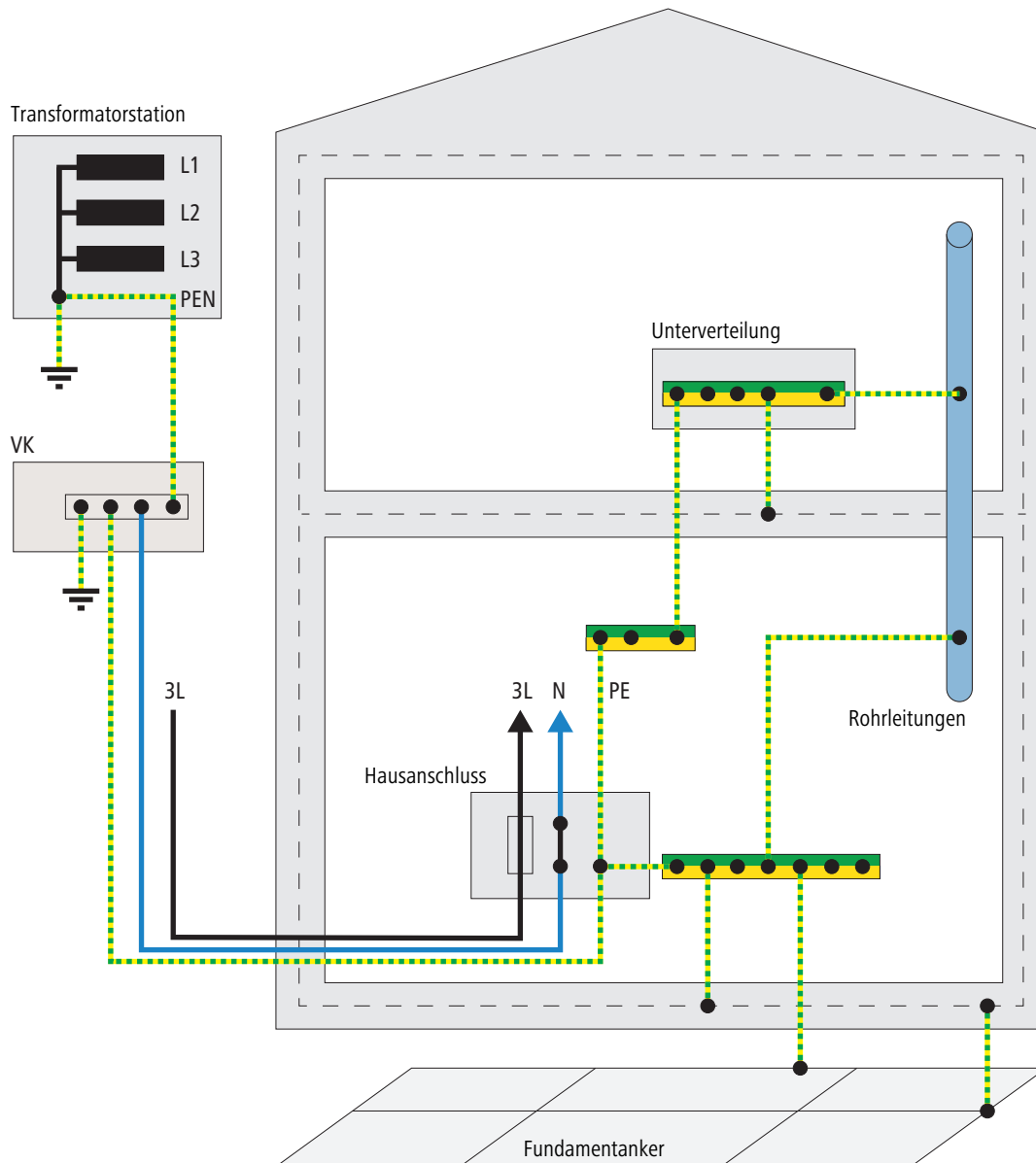
Abb. 28: TN-S-Netzsystem
