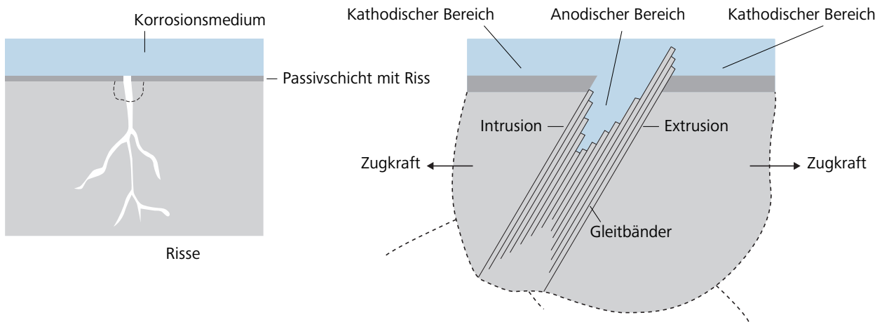
Abb. 16: Spannungsrisskorrosion
