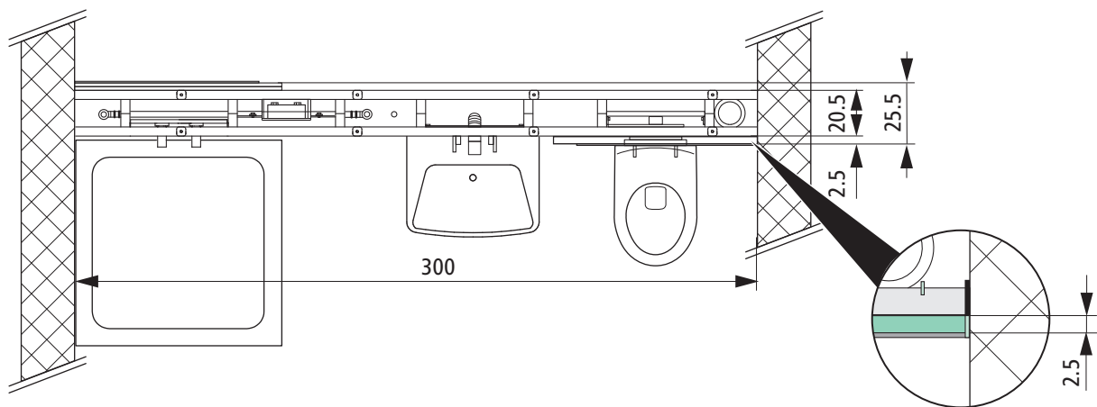
Fig. 21: Plan d'ensemble
