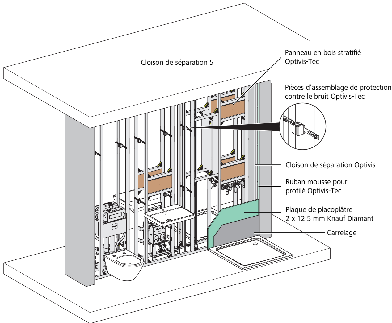
Fig. 32: Cloison de séparation Optimis 34.5 cm, équipement et carrelage sur deux côtés
